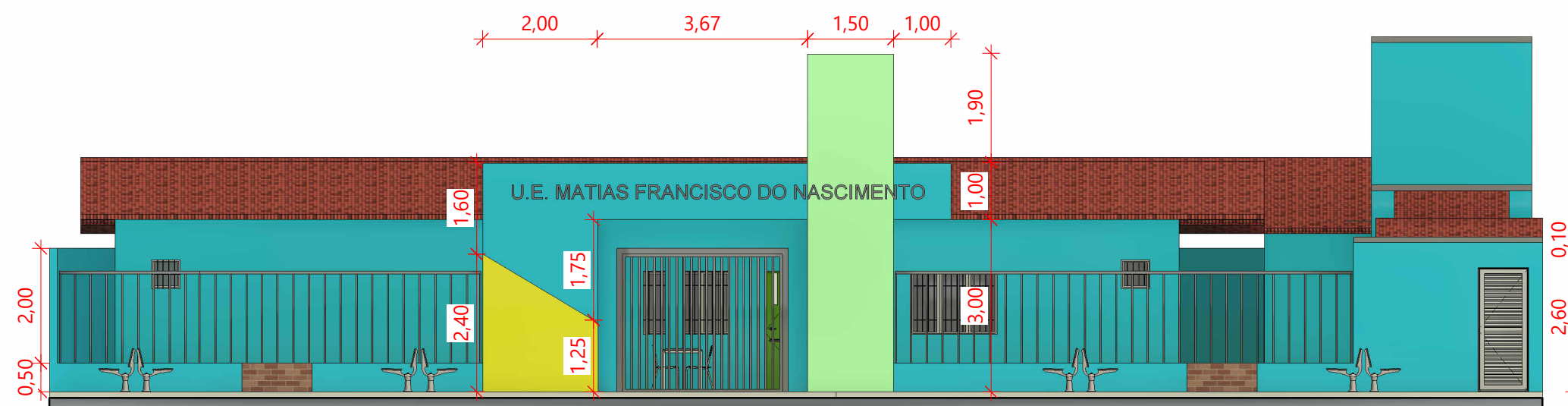
3 CORTE - FACHADA FRONTAL (MURO) ESC.: 1 : 100
