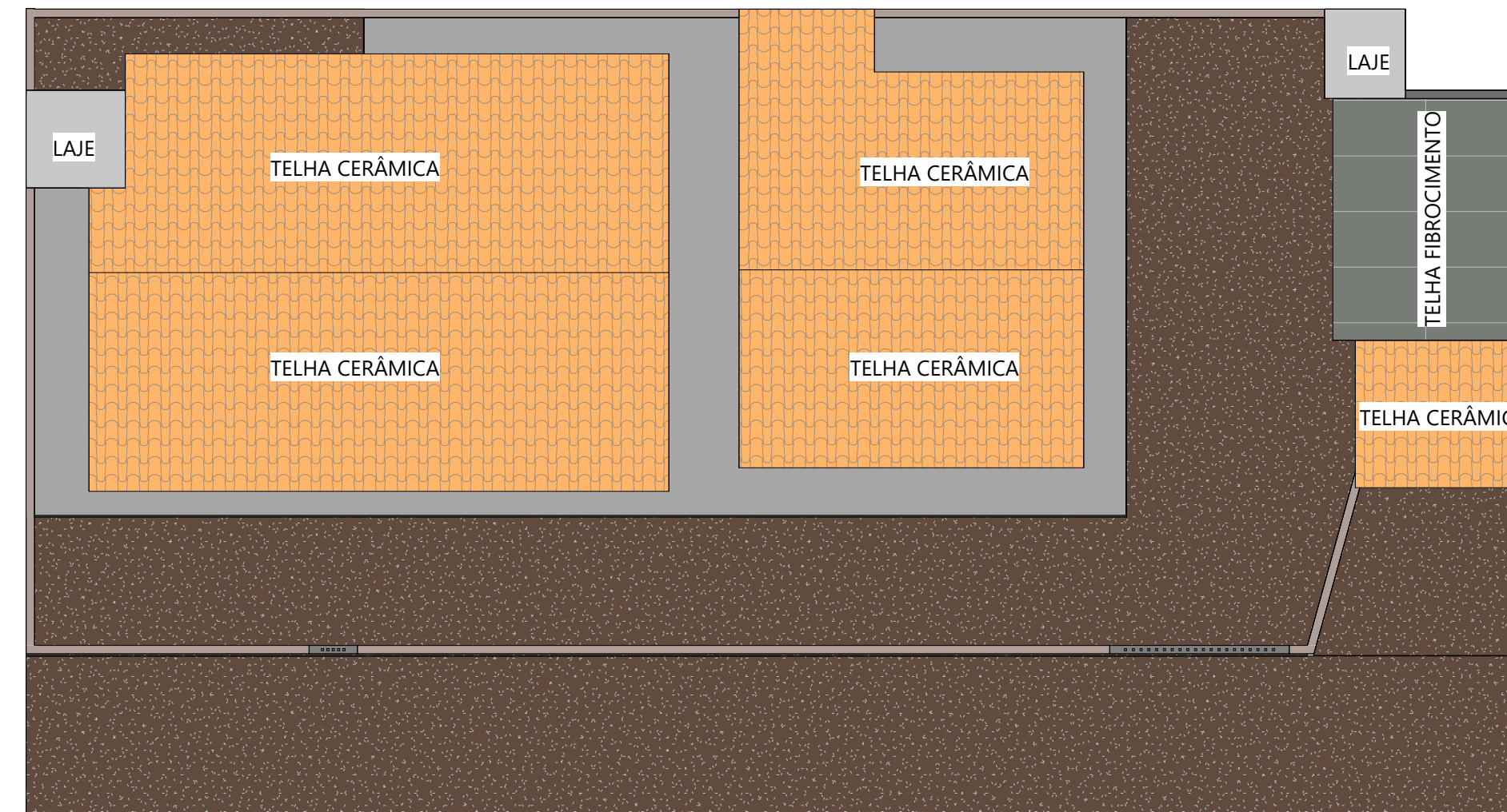
2 COBERTURA EXISTENTE ESC.: 1 : 100
