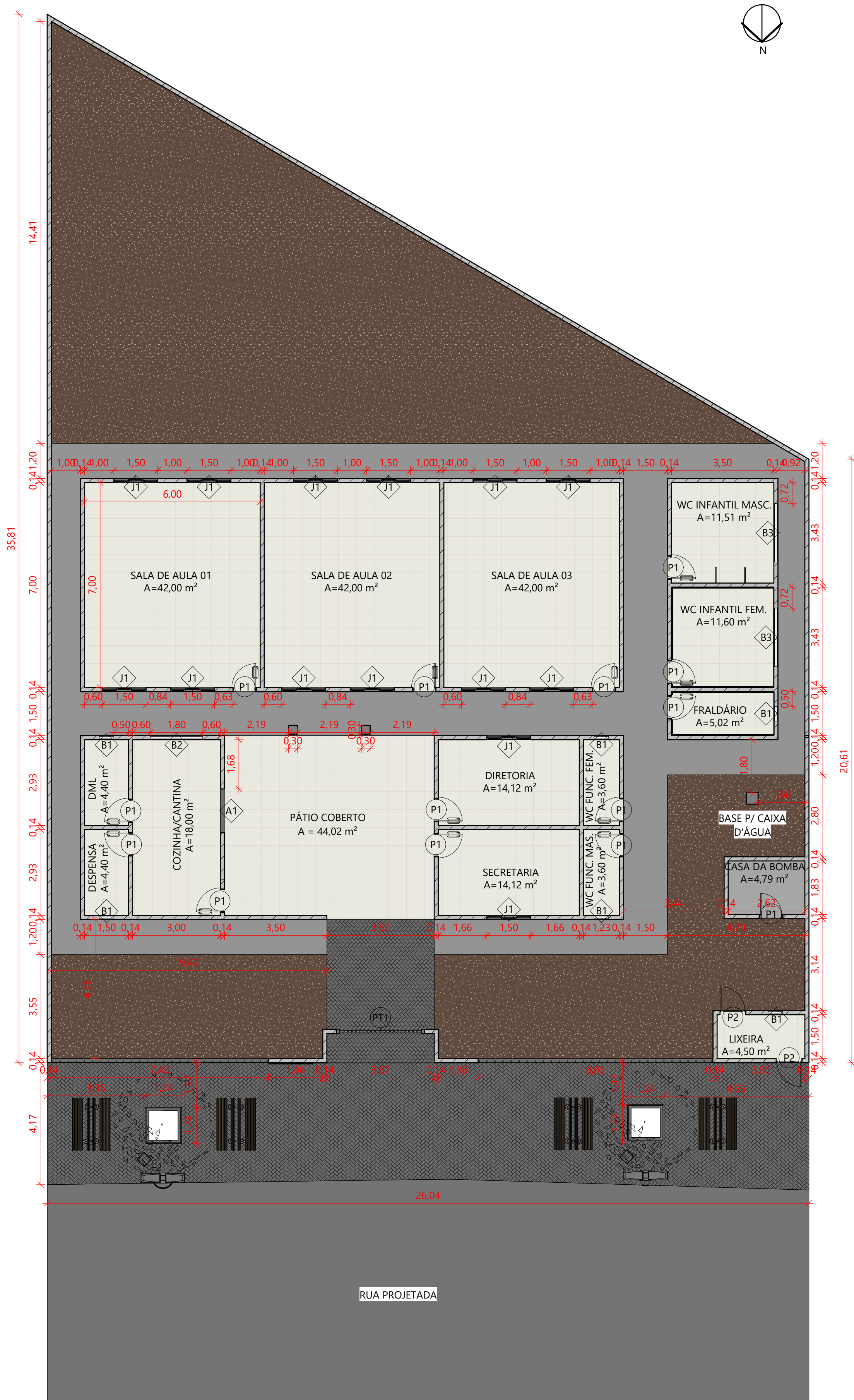
1 TÉRREO PROPOSTO ESC.: 1 : 100
