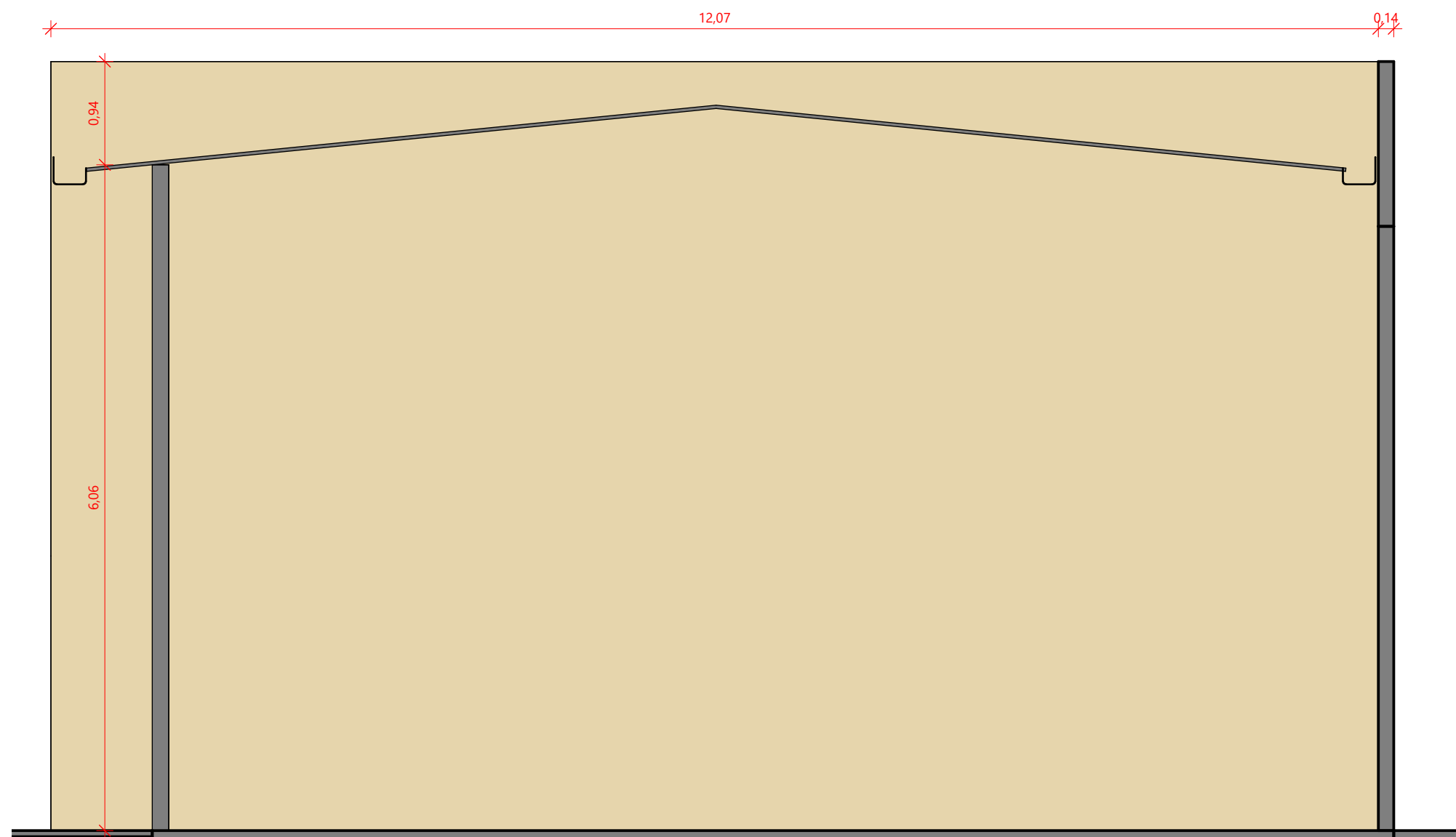
1 PÁTIO - LATERAL 1 ESC.: 1 : 50
