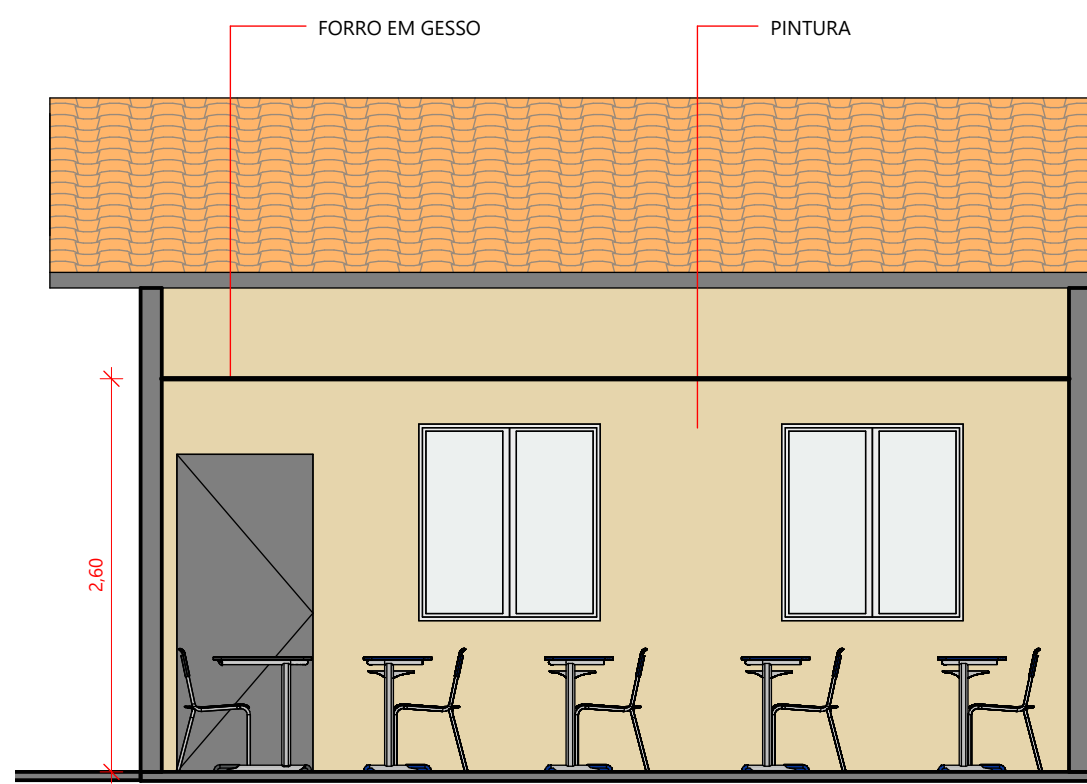
4 DETALHAMENTO - SALAS DE AULA ESC.: 1 : 50
