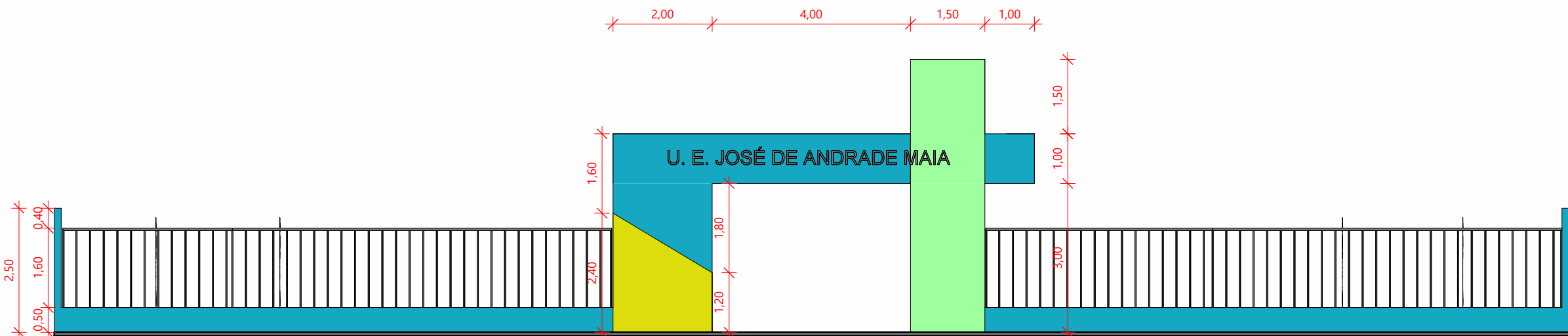
2 FACHADA FRONTAL (MURO) ESC.: 1 : 100
