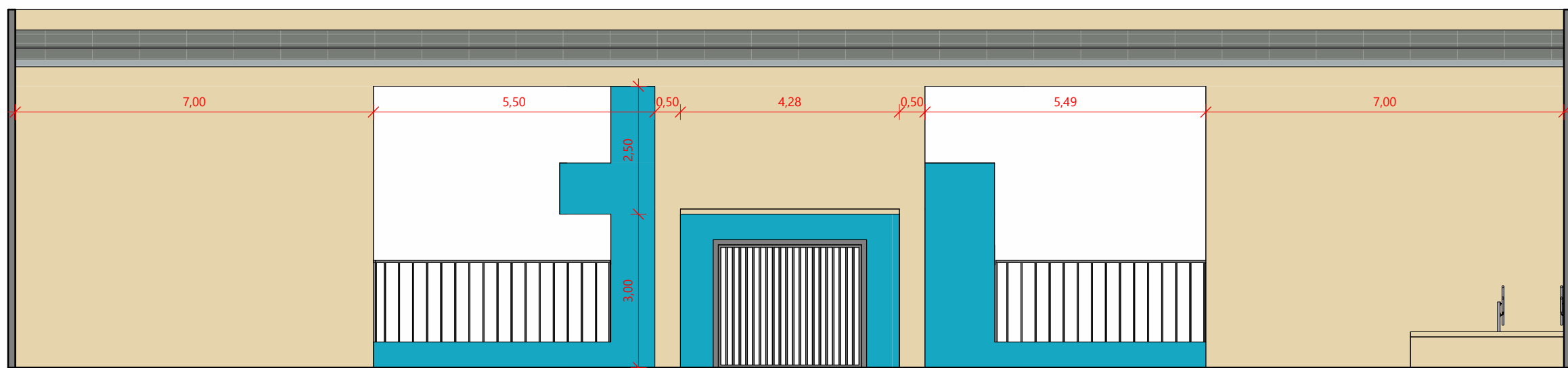
4 FACHADA/PÁTIO ESC.: 1 : 100
