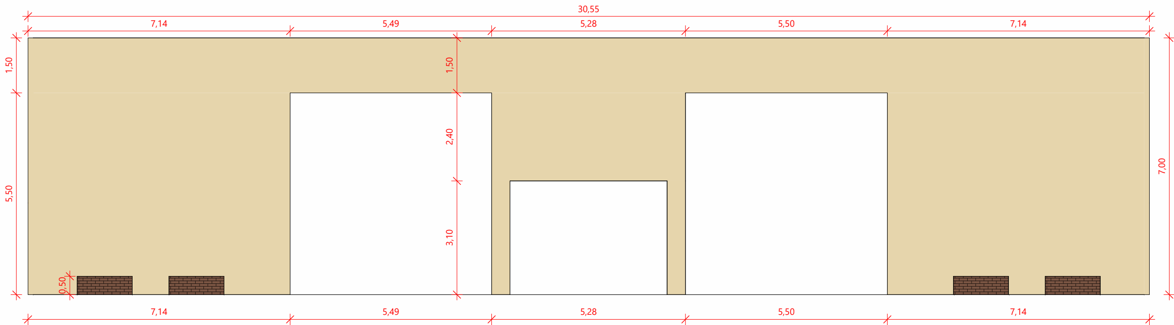
3 FACHADA FRONTAL ESC.: 1 : 100
