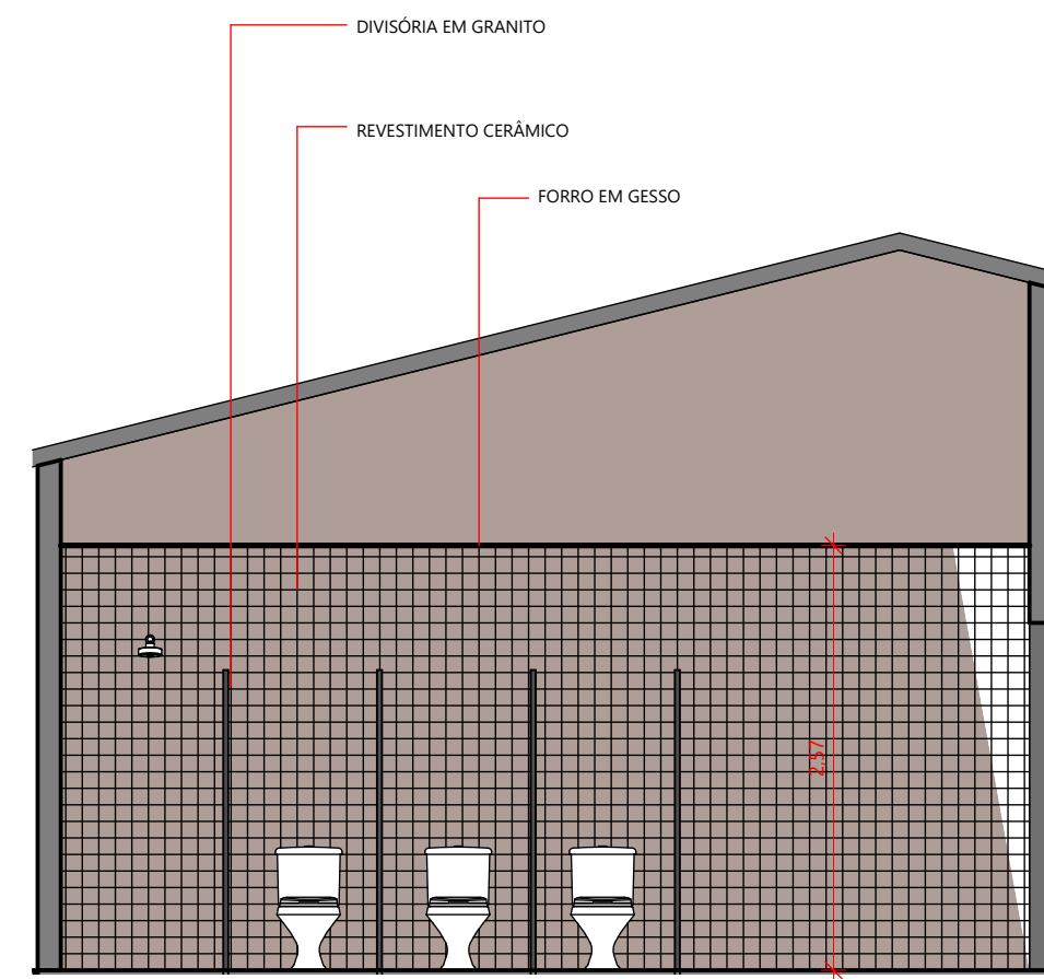
5 DETALHAMENTO - BWC ESC.: 1 : 50
